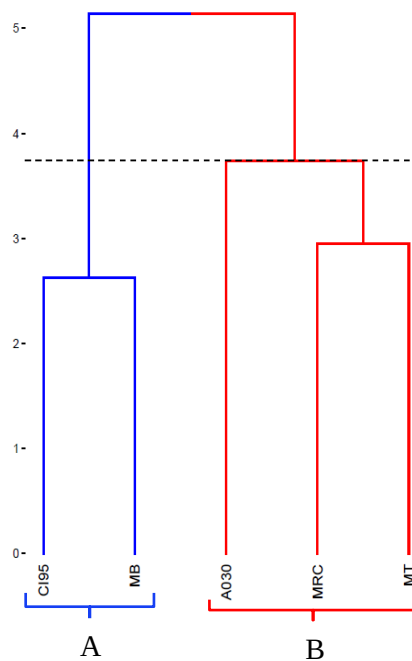
Figura 2. Agrupamiento jerárquico con distancia Euclidiana para descriptores morfo-agronómicos de cinco accesiones de maní del Banco de Germoplasma del INIA, Perú.
