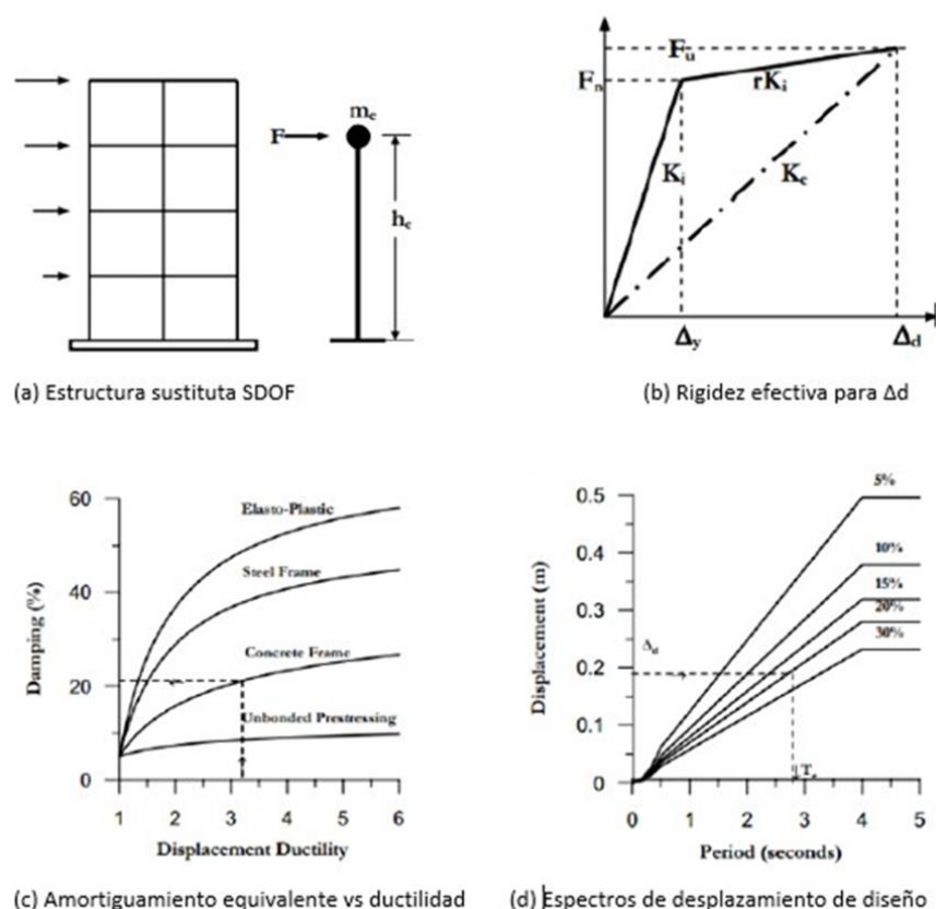
Figura 2. Proceso del Método DDBD. Fuente: [1]
