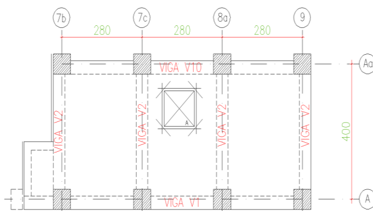
Figura 3. Losa de Mezzanine de nivel 8.00
