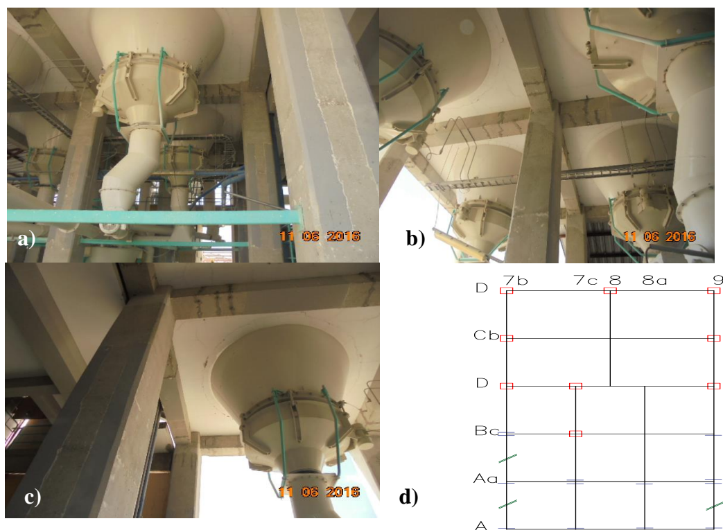
Figura 8. Daño en elementos estructurales del segundo piso alto de Silos de Harina.
