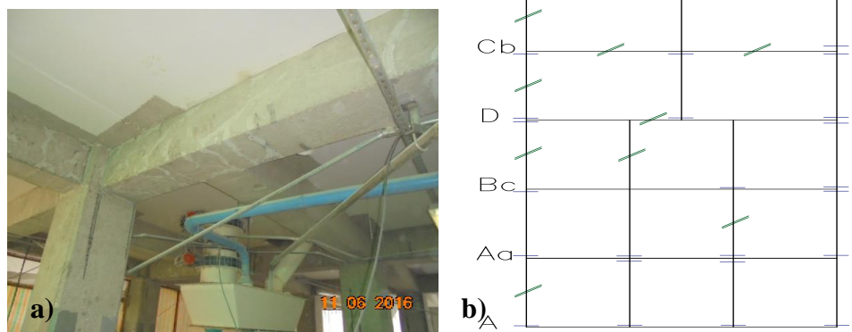
Figura 7a y 7b. Daño en vigas de primer piso alto, de Silos de Harina. Nivel 3.50 m. y esquema de fisuras Se aprecia que se ha inyectado SIKADUR 52 previa la colocación del adhesivo SIKADUR 31; la inyección ingresa en todas las fisuras por más pequeña que ésta sea, debido a que es un líquido que al secarse seca tiene resistencias muy altas. El piso que más daño sufrió durante el 16 A, fue el segundo piso alto que va desde la losa del nivel 3.50 m a la losa del nivel 10,00 m. El daño se debe a dos motivos: el primero, debido a que es un piso blando por la gran altura de sus columnas (6.50 m), y el segundo que al deformarse lateralmente la estructura resiste un gran peso proveniente de los muros de hormigón armado y harina de los silos. En la Figura 8 a, b y c, se observa que las vigas de la losa del nivel 10,00 m han sido inyectadas SIKADUR 52.
