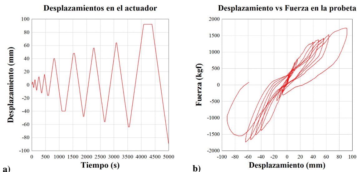
Figura 6. a) Historia de desplazamientos, b) Histéresis de la probeta. Fuente [1]
